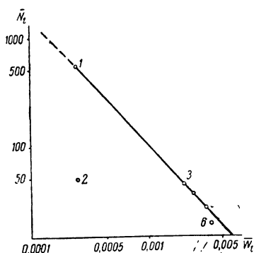
Рис. 4.3.4. Зависимость между численностью ( N_t ) и средним весом ( w_t ) личинки Tanytarsus jucundus в озере Сугарлоф. Логарифмические шкалы.
