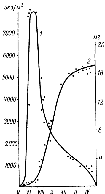
Рис. 4.2.1. Изменения плотности населения одного поколения Pontoporeia и ее рост в реке.
