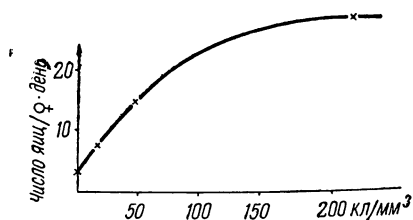
Рис. 3.3.6. Среднее число яиц, отложенных за день самкой Calanus , при различных концентрациях Chlamydomonas sp. (Marshall and Orr, 1952)
