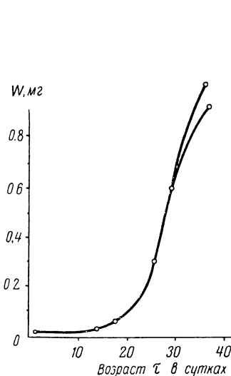
Рис. 5.3.1. Рост Calanus helgolandicus (Петипа, 1965).
