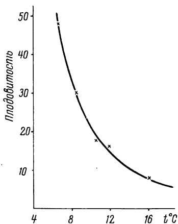
Рис. 3.3.3. Отношение между плодовитостью и температурой у Pseudocalanus (построен на основании рисунков 3.3.1 и 3.3.2).
