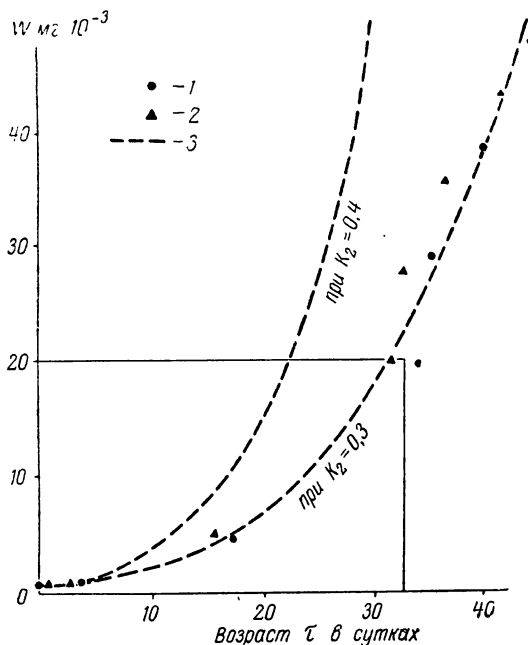
Рис. 5.3.5. Рост особей в популяции Cyclopidae с учетом продукции яиц в белорусских озерах в среднем за сезон (с мая по октябрь) (Шушкина, 1965). 1 и 2 — эмпирические данные по росту Cyclopidae в озере Мясро (1) и озере Баторно (2), 3 — теоретические кривые роста при Q = 0,165w^{0,8} , K_2 = 0,4 и 0,3 .
