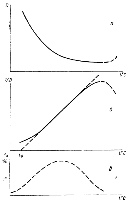
Рис. 3.2.1. Общий вид зависимости от температуры:
