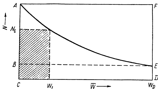
Рис. 4.3.3. Схематический график зависимости между численностью ( \bar{N}_t ) и средним весом одной личинки ( \bar{w} ). (См. текст, Nees and Dugdall, 1959.)
