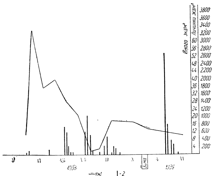
Рис. 1. Динамика численности личиночных и имагинальных стадий Chironomus plumosus в озере Малое Медвежье:
