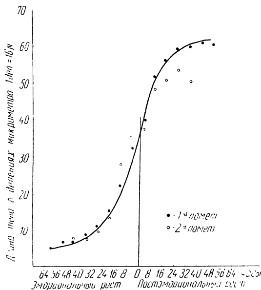
Рис. 1 Линейный рост аспланхны из озера Дривяты в лабораторных условиях.
