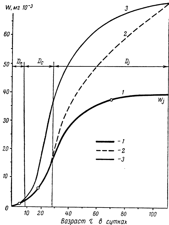
Рис. 5.3.7. Рост Acartia clausi по данным В. Н. Греза (1964). 1 — кривая В. Н. Греза без учета продукции яиц, 2 — та же кривая с учетом продукции яиц, 3 — исправленная кривая.
