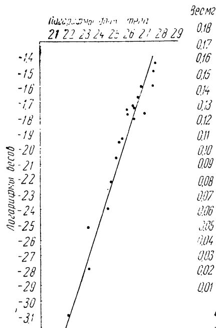
Рис. 2. Зависимость между логарифмами длины и веса тела (мг) аспланхны.
