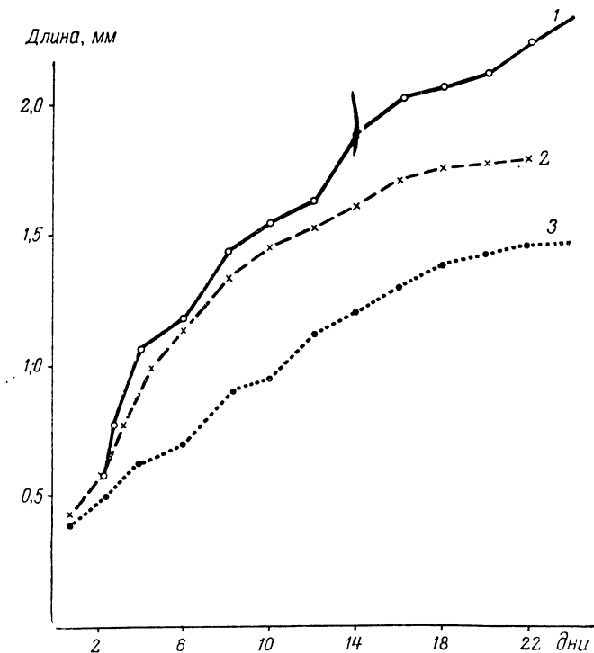
Рис. 3.3.4. Рост Daphnia galeata mendotae на разных концентрациях пищи (Hall, 1964).
