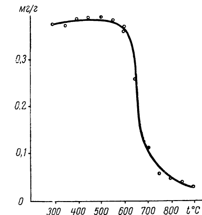
Рис. 2.2.1. Содержание калия в золе в зависимости от температуры прокаливания проб в муфельной печи (Grove et al., 1960).
