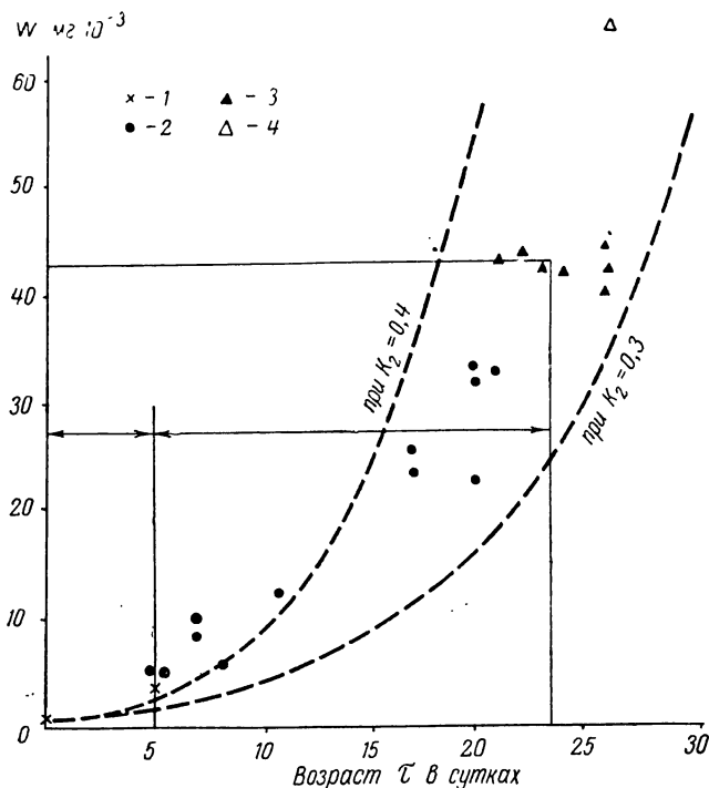
Рис. 5.3.4. Рост Macrocyclus albidus при t = 21^\circ \text{C} и концентрации инфузорного корма 1 \text{ г/м}^3 (Клековский, Шушкина, в печати). 1 — науплиусы, 2 — копеподиты, 3 — взрослые, 4 — прирост взрослого рачка за счет образования яиц первой кладки (1 и 2 — кривые роста, рассчитанные по уравнению 5.3.5, при K_2 = 0,4 и 0,3 и Q = 0,165\omega^{0,8} ).
