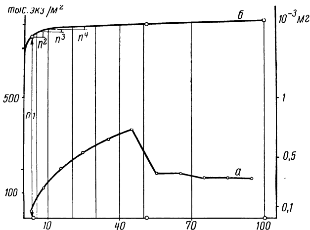
Рис. 3. Расчет продукции Epischura baicalensis графическим методом В. Н. Грезе. Численность и интенсивность прироста: а — кривая темпа прироста одной особи в зависимости от ее веса (на оси абсцисс — вес особи в 10^{-3} мг, а на оси ординат — суточный прирост в 10^{-3} мг); б — кривая зависимости численности от веса (на оси абсцисс — максимальный вес науплиусов, копеподитов и взрослых с учетом продукции их яиц, на оси ординат — нарастающим итогом численность науплиусов, копеподитов и взрослых в тысячах экземпляров на кв. метр, n_1, n_2, \dots, n_n — количество особей, имеющих вес в пределах, ограниченных соседними вертикалями в тысячах экземпляров на кв. метр).
