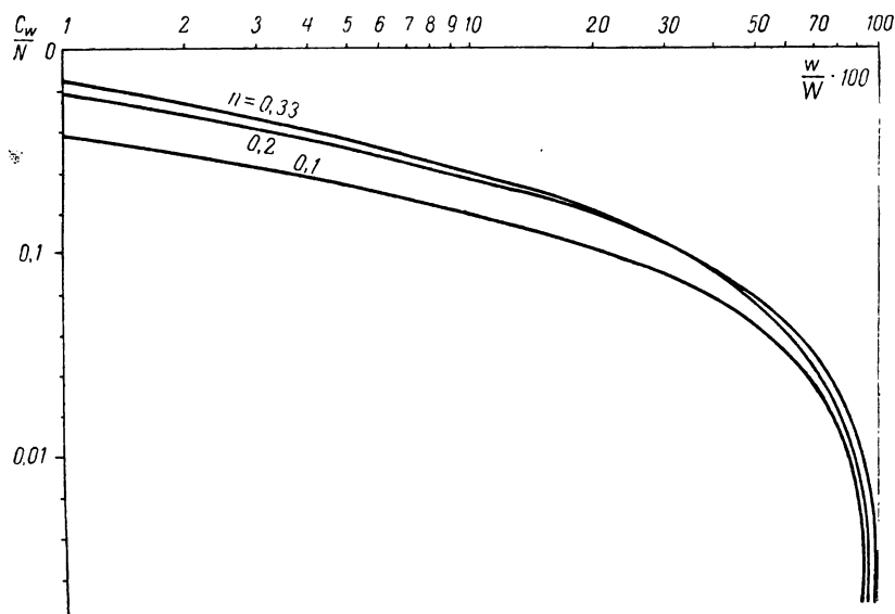
Рис. 3.1.4. Зависимость между удельной скоростью роста C_w и константой N по уравнению (3.1.12a) при трех разных значениях n .
