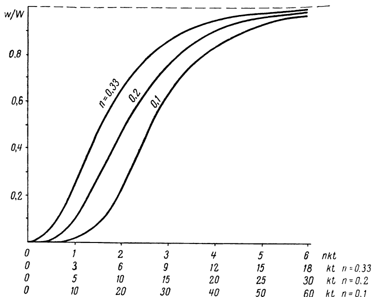
Рис. 3.1.3. Кривые роста, построенные по уравнению (3.1.126), при трех различных значениях n .
