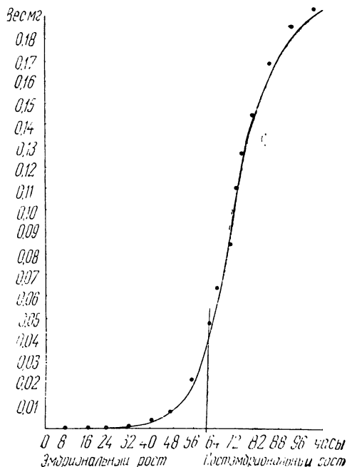
Рис. 3. Весовой рост аспланхны в лабораторных условиях (по наблюдениям за особями первого помета от самок, взятых из озера Дривяты).
