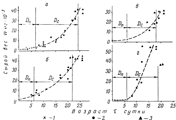
Рис. 5.3.3. Рост Macrocyclus albidus при разных концентрациях корма (Клековский, Шушкина, 1966).
