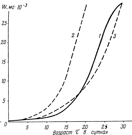
Рис. 5.3.2. Рост Acartia clausi . 1 — кривая по эмпирическим данным Т. С. Петипа (1965), 2 — теоретическая кривая параболического роста при M = 0,437 и K_2 = 0,2 (Петипа, 1965), 3 — теоретическая кривая параболического роста при M = 0,300 и K_2 = 0,2 .
