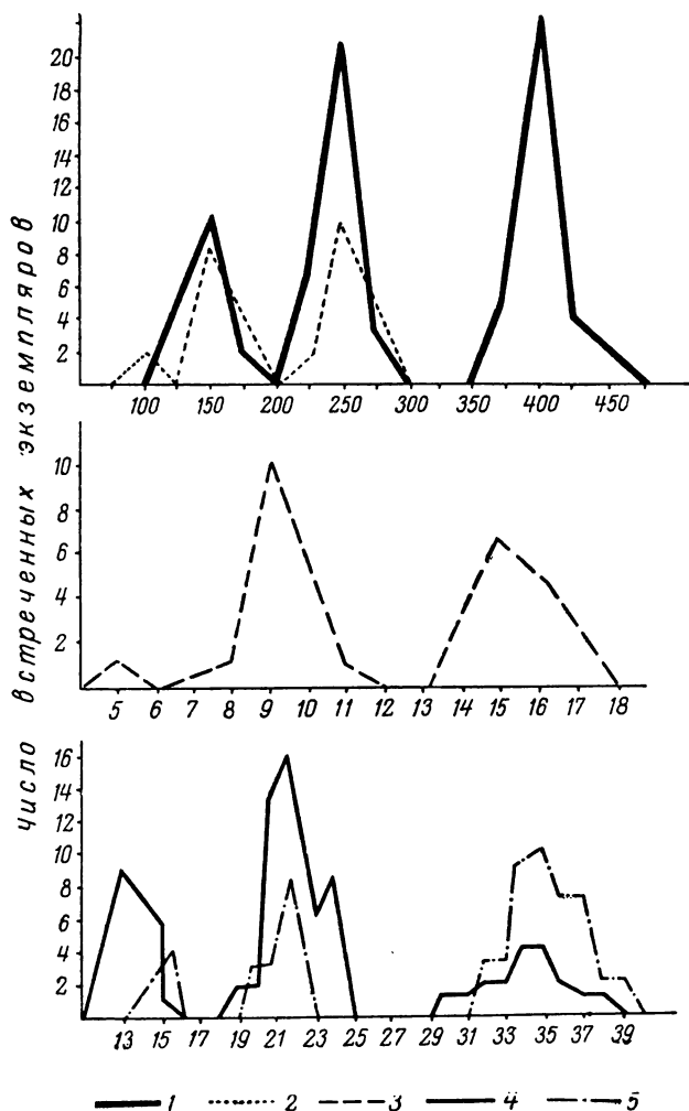
Рис. 4.3.2. Ширина головных капсул у личинок Polypedilum gr. nubeculosum (1), Tanytarsus gr. manicus (2), Cricotopus gr. silvestris (3), Procladius sp. (4), Anatopinia gr. varia (5) (Константинов, 1951). По оси абсцисс — ширина головной капсулы в \mu (для 1 и 2) и в делениях окуляр-микрометра (3, 4, 5)
